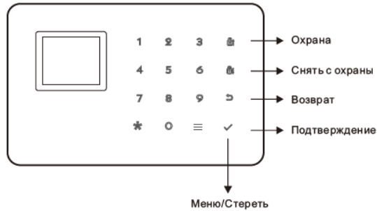
Рисунок 2. Контрольная панель. Вид сбоку.
